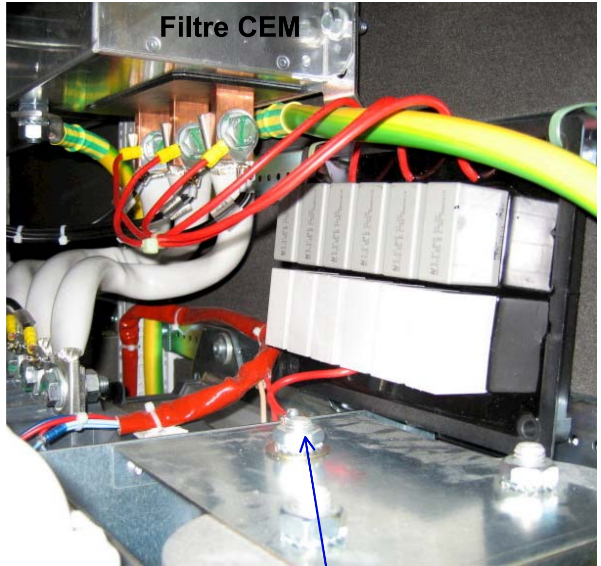
Meilleur câblage (malgré des fils trop longs)
